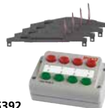
55392 Weichenantrieb-Set 99,99 €* Dieses Set enthält 1 mal das Stellpult # 55262 zum Schalten von Weichen oder Signalen und 4 mal den elektrischen Weichenantrieb # 55271 für alle Weichen.
