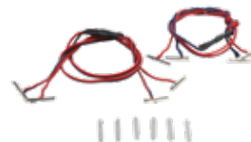
55391 Kehrschleifengarnitur 14,10 €* Kehrschleifengarnitur zum problemlosen Befahren von Kehrschleifen. Bestehend aus Isolierverbindern, Kabeln und Anschlussverbindern. Nicht einsetzbar für Digital-Betrieb.
